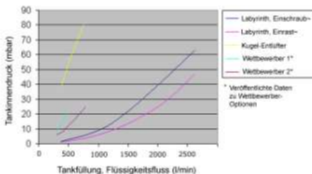
Labyrinth-Entlüfter – Leistungsvergleich
