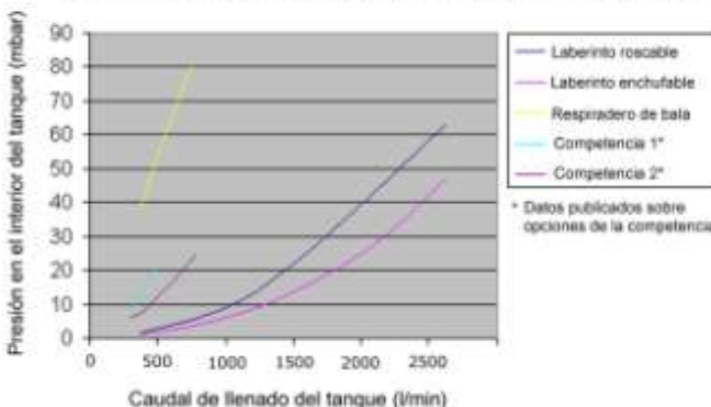
Comparación del desempeño del respiradero en laberinto
