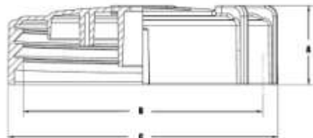
Dimensiones estándar de la tapa para tanques rosca hembra
